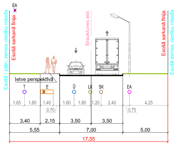
Šķēršprofils 3-3 (Eduarda Veidenbauma iela)
