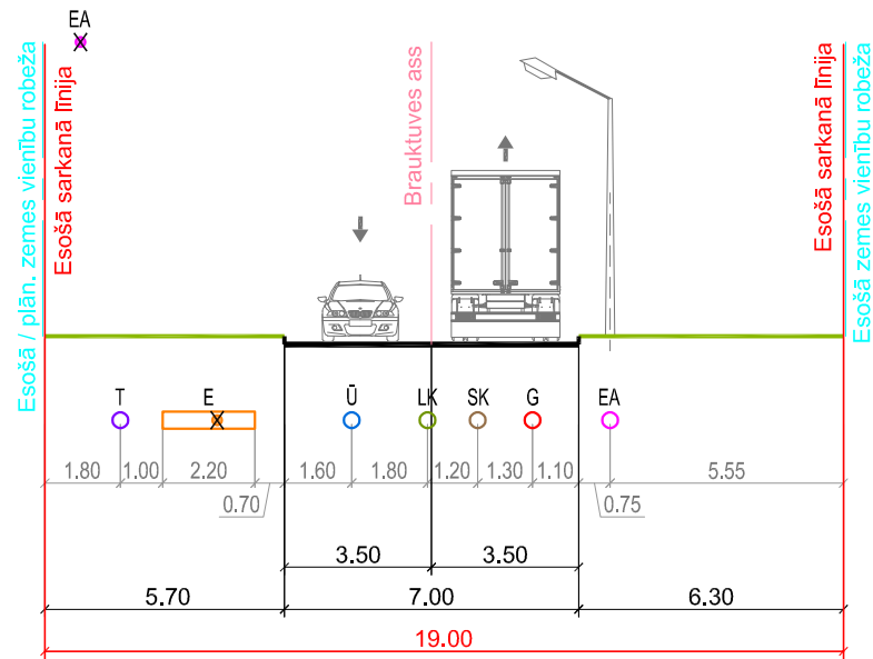
Šķēršprofils 2-2 (Eduarda Veidenbauma iela)
