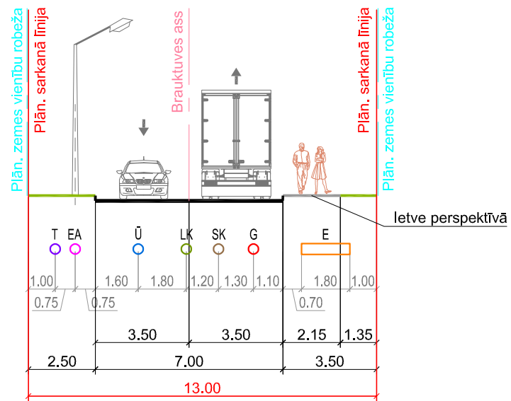
Šķēršprofils 1-1 (plānotā iela)
