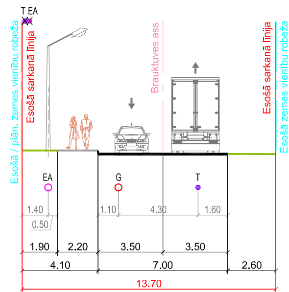
Šķēršprofils 4-4 (Robežu iela)
