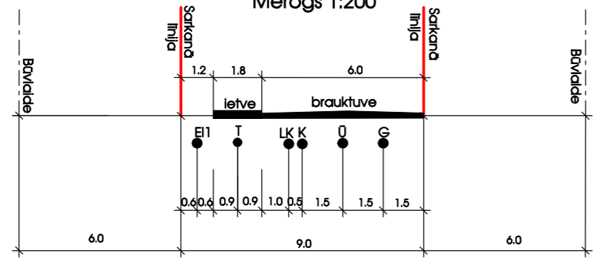
IELAS PROFILS A-A Mērogs 1:200
