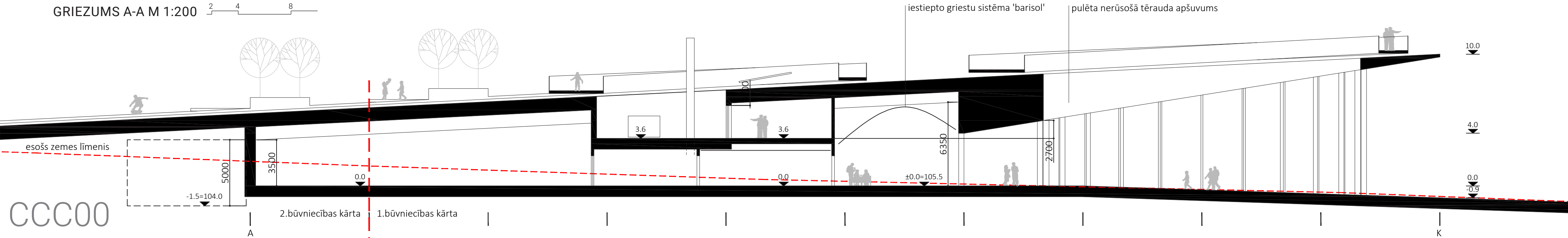
GRIEZUMS A-A M 1:200
